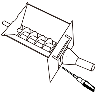
<채프 처리기 헤드 분리 전>
