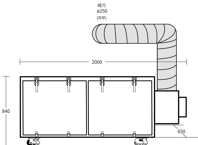
< 제연기 >
